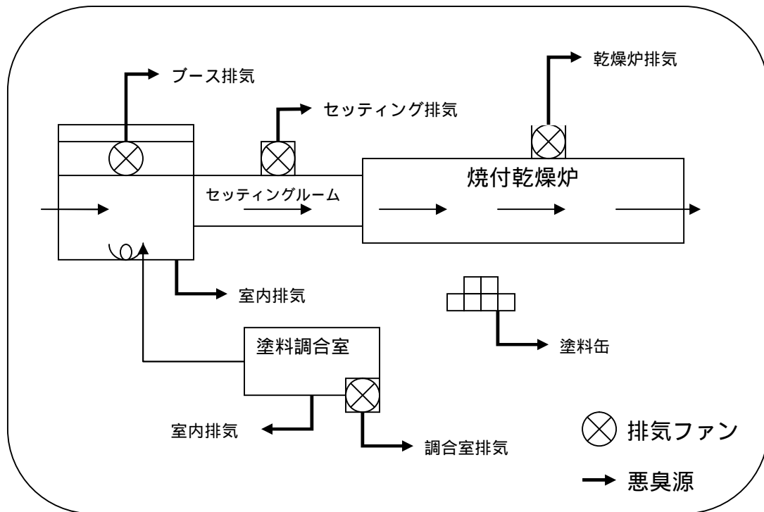
図 1 . 塗装工場における悪臭の予想される箇所
